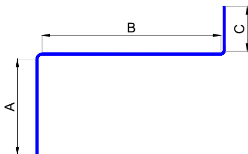
KEY: 5 - Zakladací profil pre predsadenie panelu
