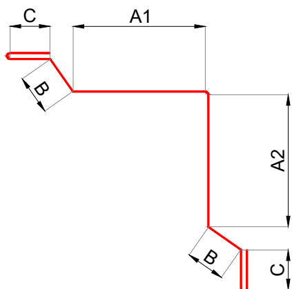
KEY: 2 - Rohová lišta
