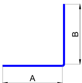
KEY: 5 - Zakladací profil pre predsadenie panelu
