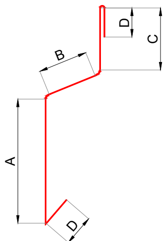
KEY: 2 - Odkvapová lišta okna
